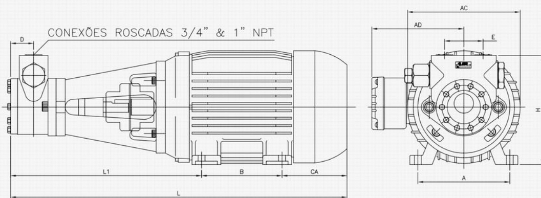
CORTE A-A
